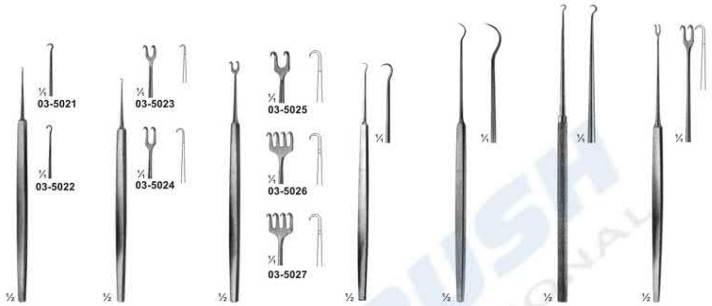
03-5021 - 03-5022 03-5021 Sharp 03-5022 Blunt GRAEFE 125 mm 03-5023 - 03-5024 03-5023 125 mm 03-5024 130 mm Sharp GUTHRIE 03-5025 - 03-5027 03-5025 130 mm 03-5026 135 mm Sharp 03-5027 135 mm Blunt ROLLET 03-5028 FRAZIER Dura Retractor 130 mm 03-5029 TOENNIS Dura Retractor 150 mm 03-5030 KILNER 160 mm 03-5031 FREER 150 mm
